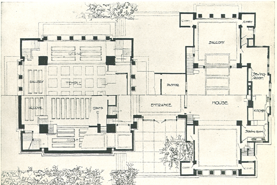
BIJLAGE VIII VAN „DE STIJL”, TWEEDE JAARGANG N o . 4. UNITY CHURCH MET PLATTEGROND (BEGANE GROND) DOOR LLOYD WRIGHT.
